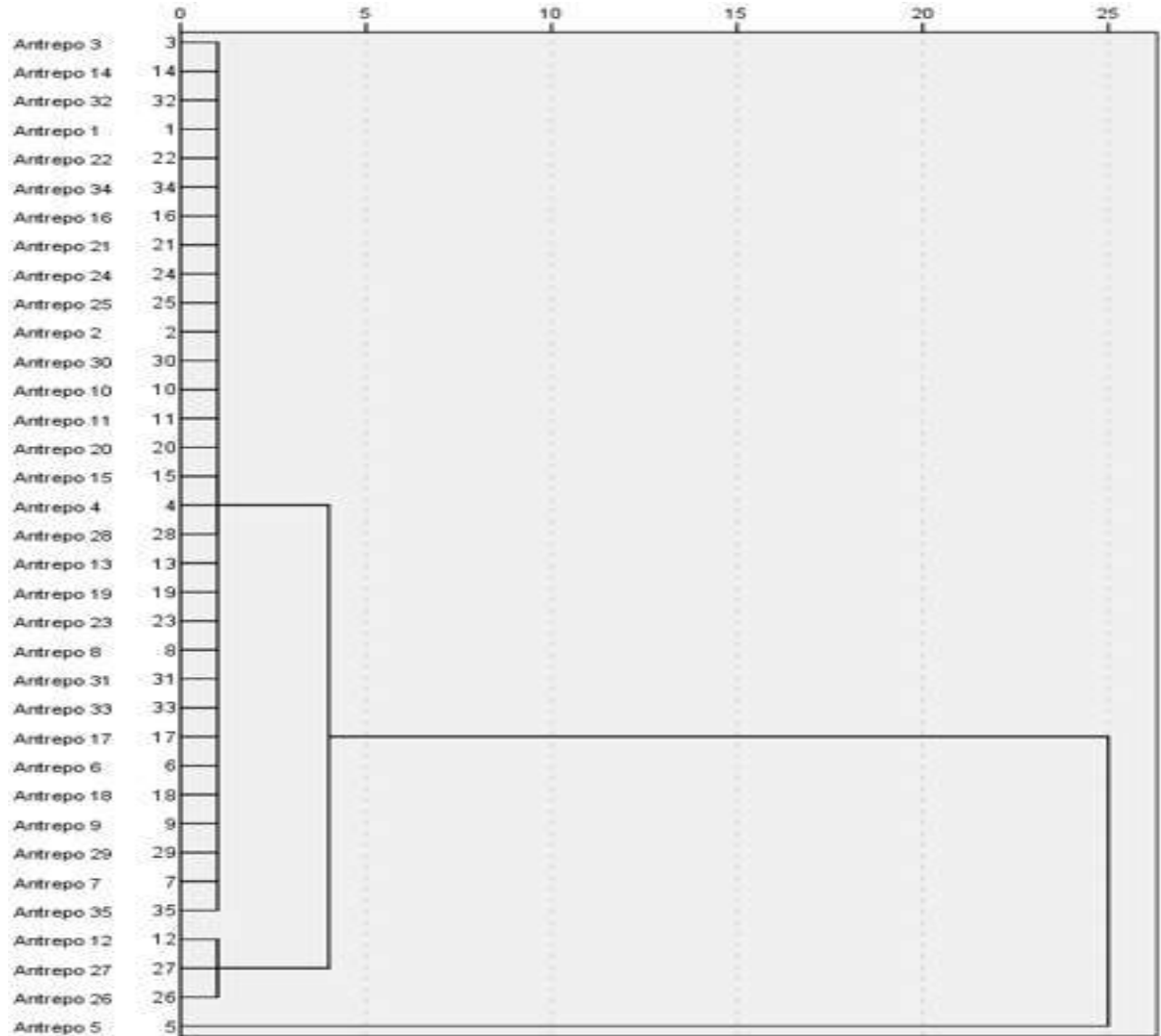
Şekil 1. Kümeleme Analizi Sonuçları
